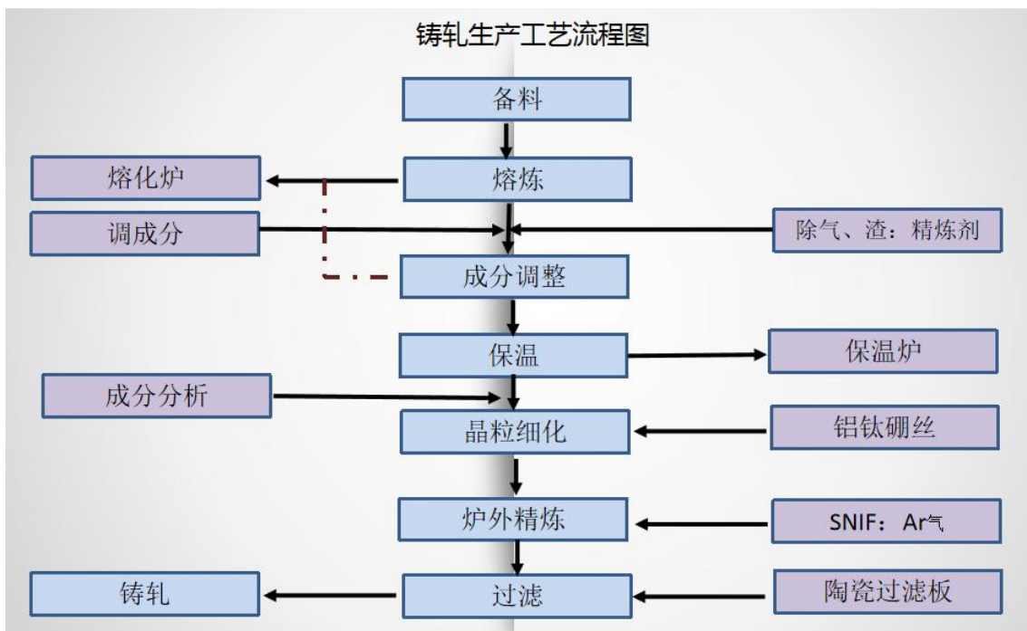
铸轧生产工艺流程图
