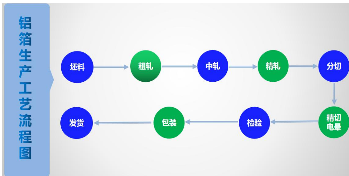
铝箔生产工艺流程图
